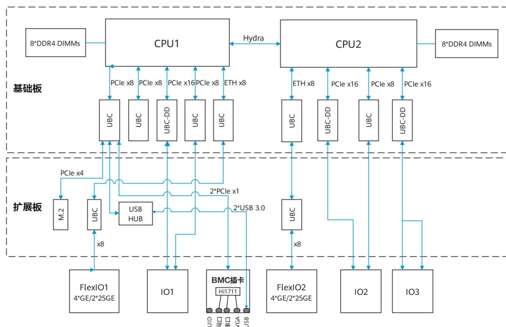
图 4-1 逻辑结构
