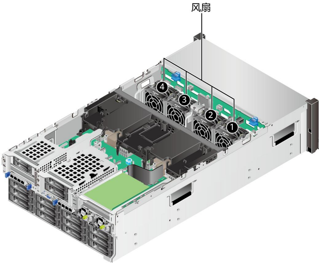
图 5-7 风扇位置图
