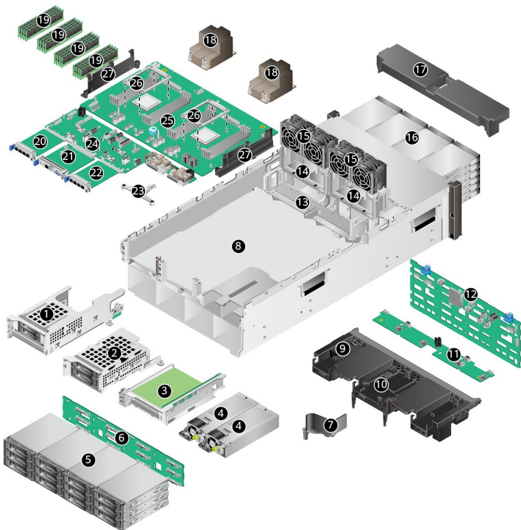
图 3-1 部件
