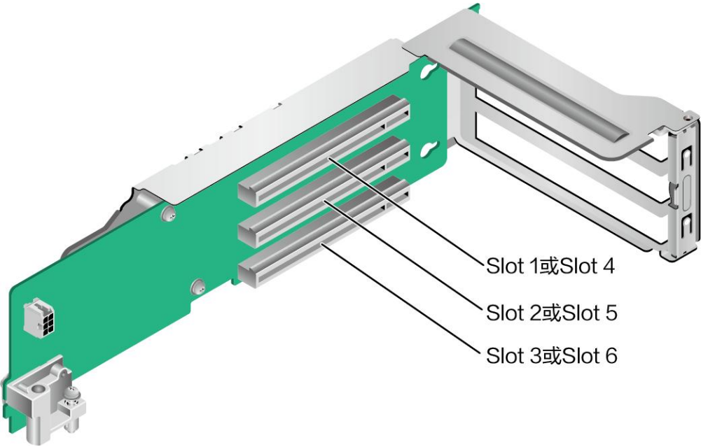
图 5-21 3*x8 Riser 卡
