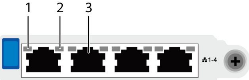
图 5-26 SF221Q（4xGE 电口）
