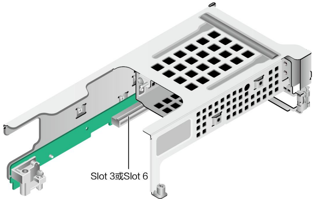
图 5-23 1*x16 Riser 卡
