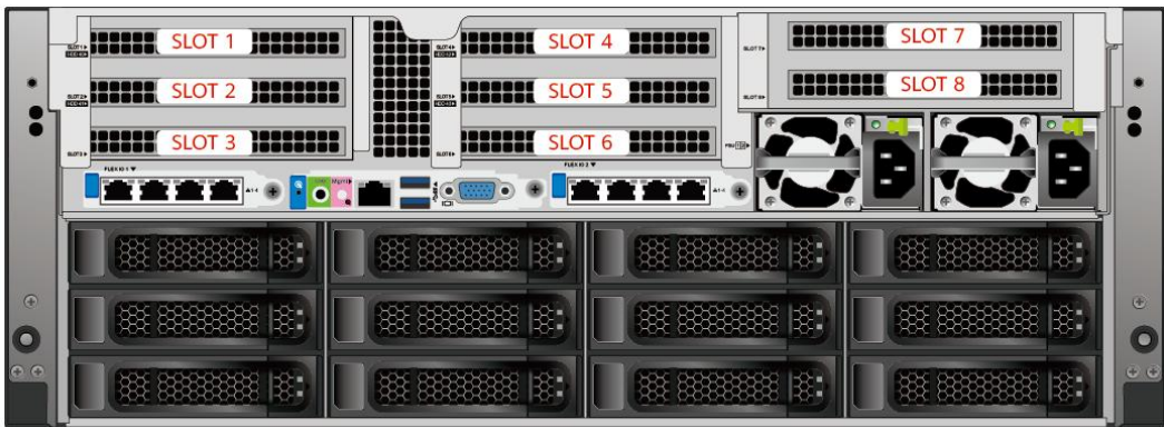
图 5-25 PCIe 插槽
