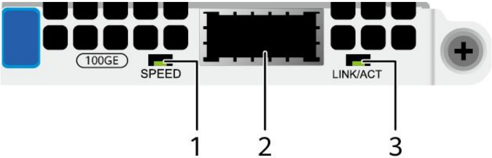
图 5-28 SF225S-H（1x100GE 光口）
