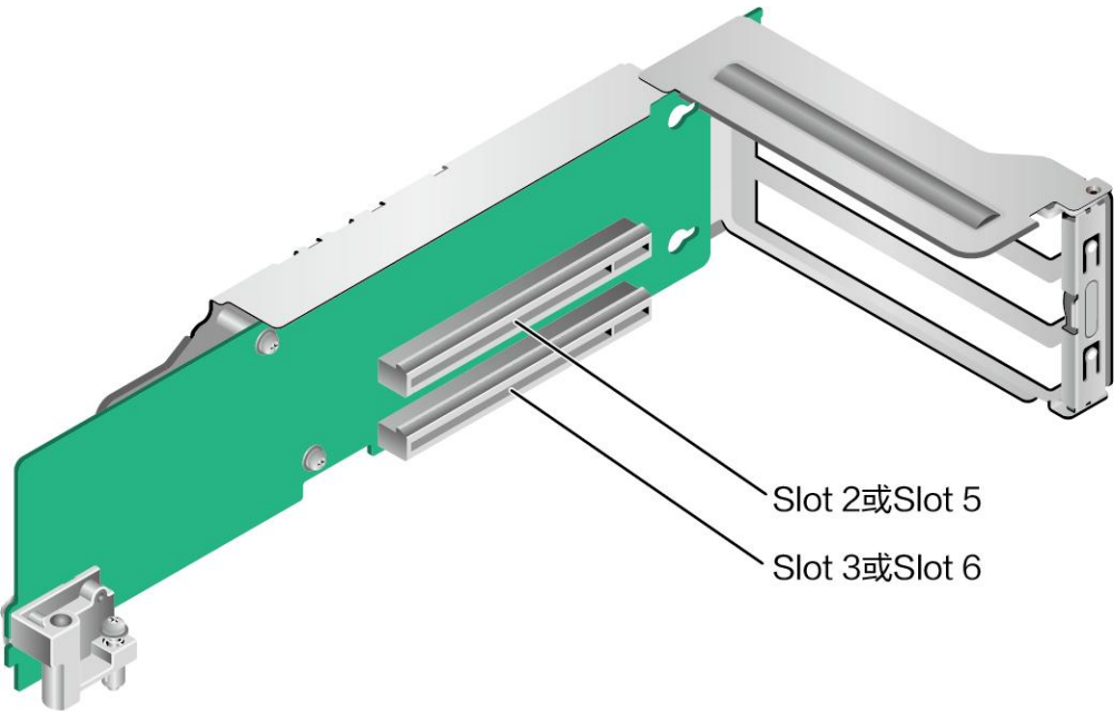
图 5-22 2*x8 Riser 卡
