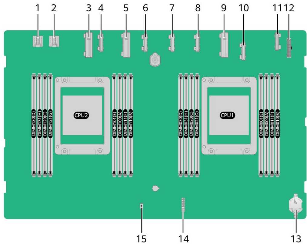
图 5-3 基础板接口
