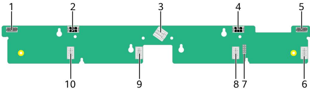
图 5-6 风扇板接口
