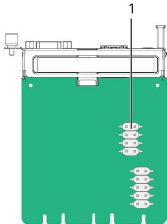
图 5-29 BMC 插卡
